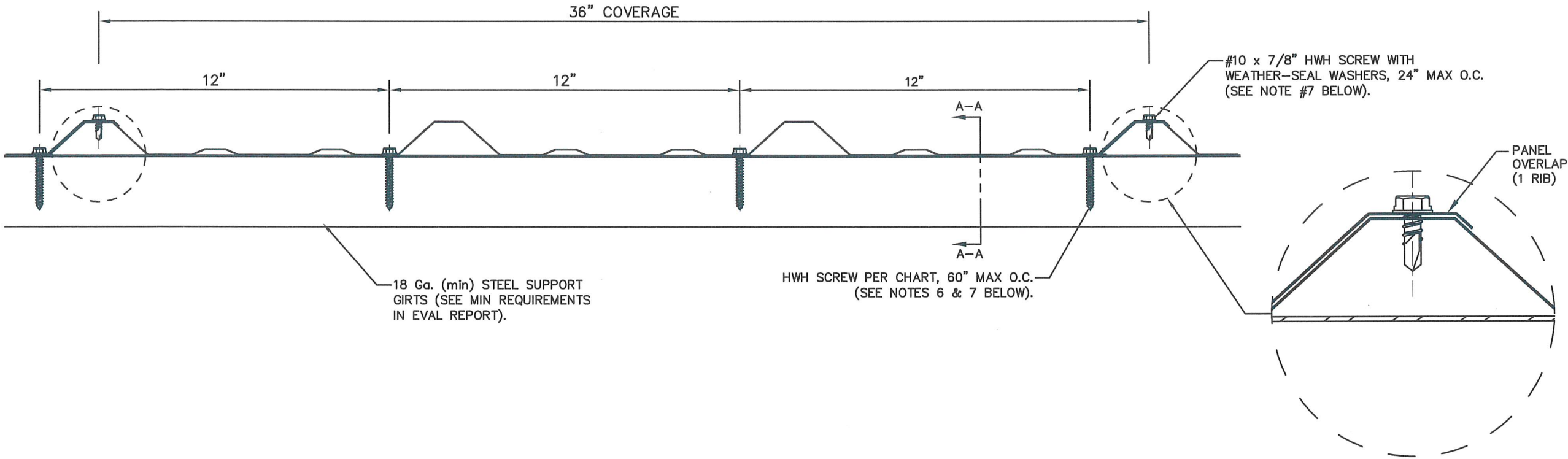
SECTION A-A
